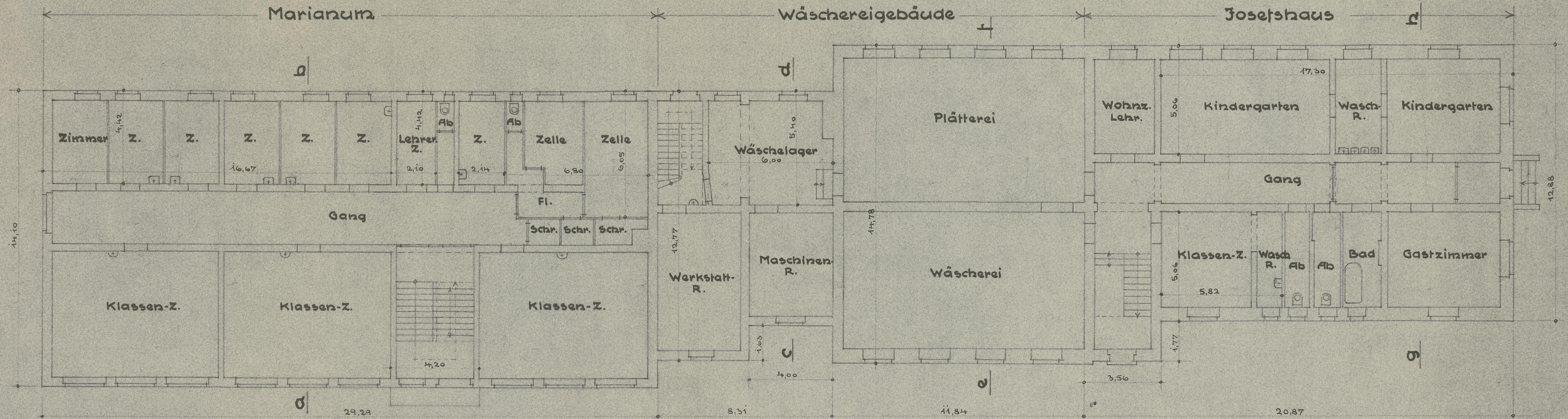
Erdgeschoßgrundriß
