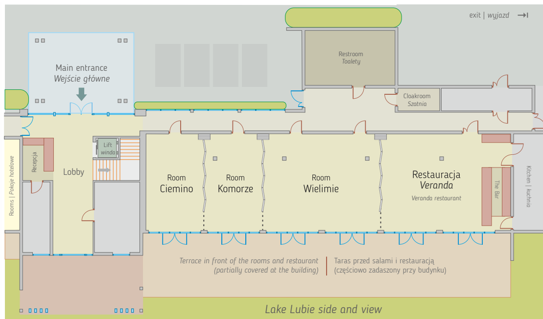
SCHEMAT KONDYGNACJI | Groundfloor plan
